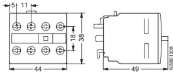
Рис.2 Габаритные размеры 3RH1921-1FA
